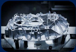
Obudowa przekładni silnika elektrycznego
